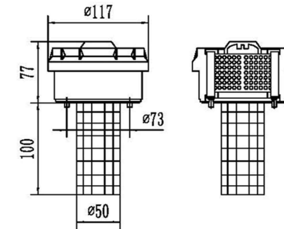
Воздушный фильтр
