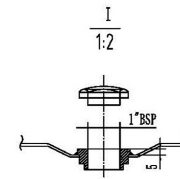
Воздушный фильтр
