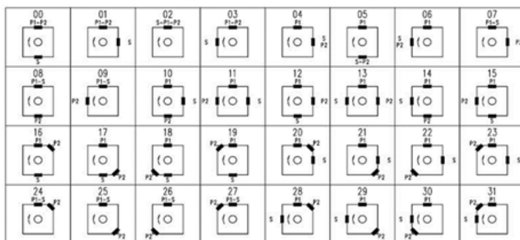
Расположение портов
